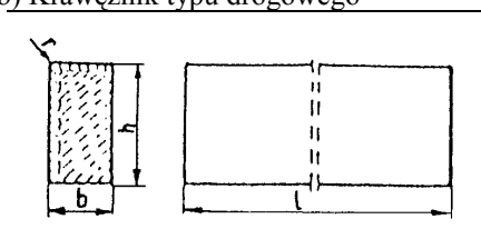
b) Krawężnik typu drogowego
