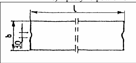
Rys. 1. Wymiarowanie krawężników
