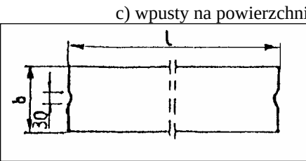
Rys. 1. Wymiarowanie krawężników
