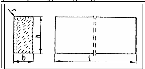
j) Krawężnik typu drogowego
