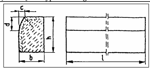
i) Krawężnik typu ulicznego
