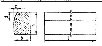
a) Krawężnik typu ulicznego
