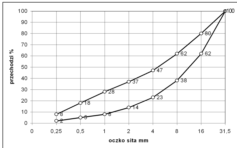
Rysunek 2. Graniczne krzywe uziarnienia kruszywa 0÷31,6 mm (dla betonu klasy B25)
