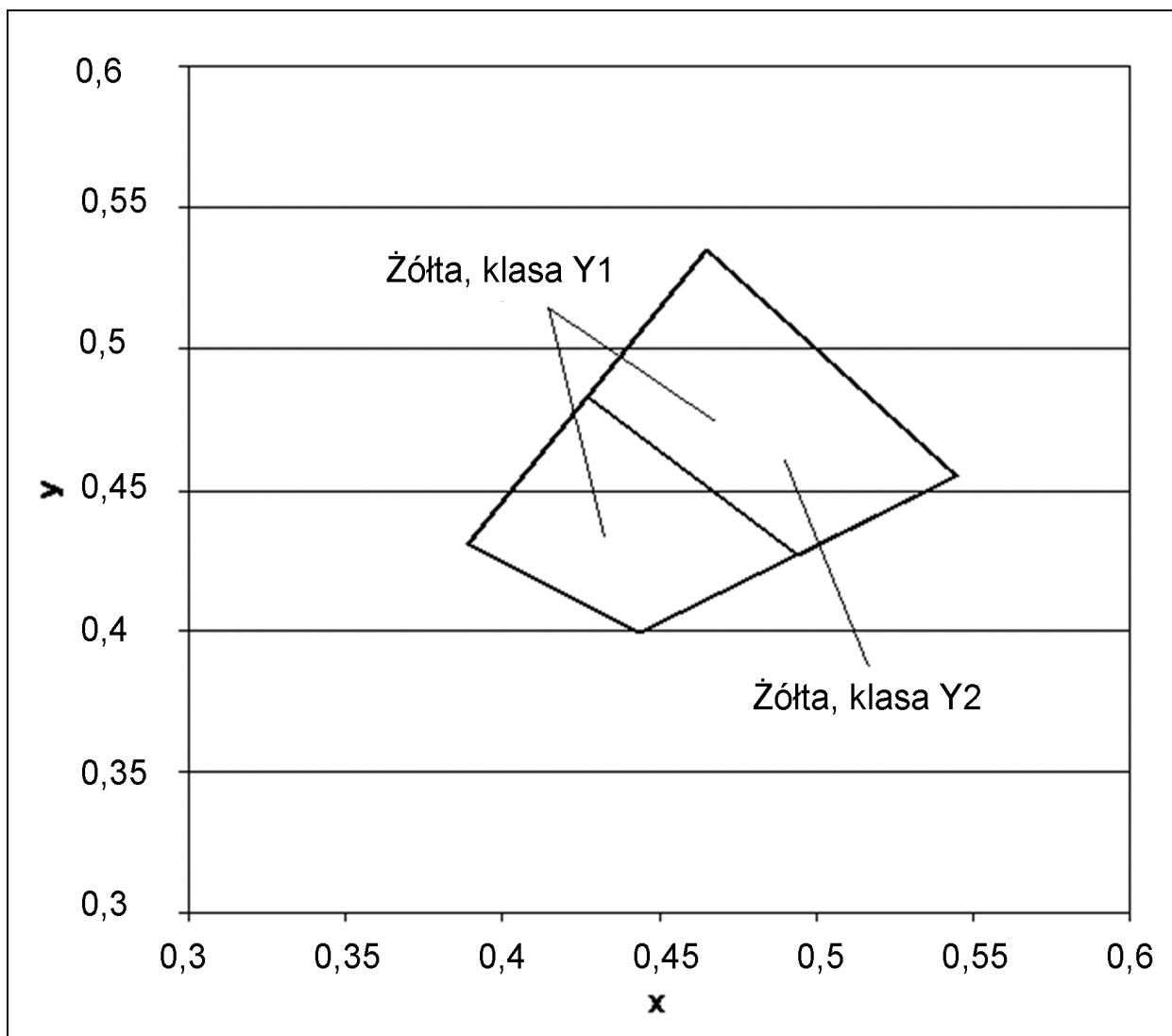
Rys.2. Współrzędne chromatyczności x,y dla barwy żółtej oznakowania
