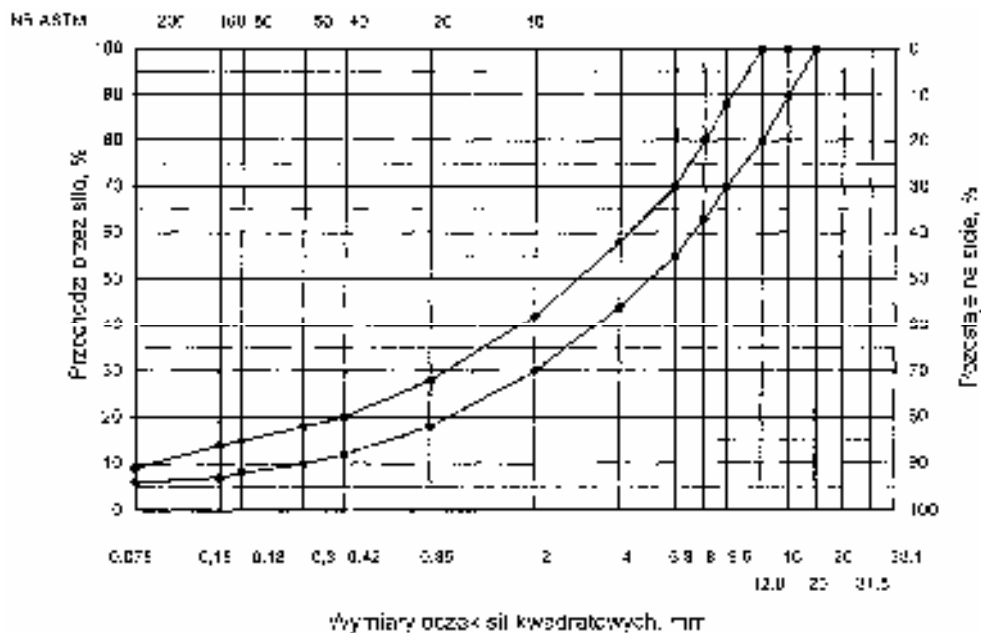
Rys. 6. Krzywe graniczne uziarnienia mieszanki mineralnej BA od 0 do 16 mm do warstwy ściernalnej nawierzchni drogi o obciążeniu ruchem od KR3 do KR6
