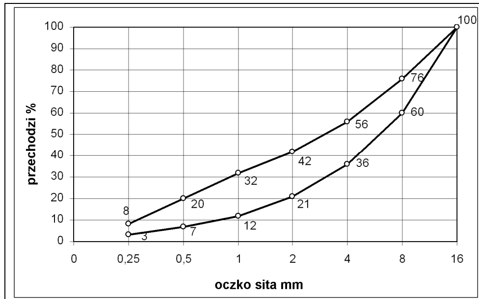
Rysunek 1. Graniczne krzywe uziarnienia kruszywa 0 ÷ 16 mm (dla betonu klasy B30)
