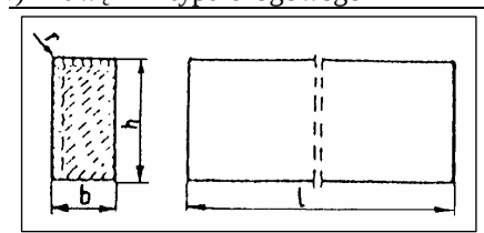
j) Krawężnik typu drogowego
