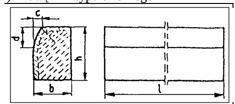
i) Krawężnik typu ulicznego
