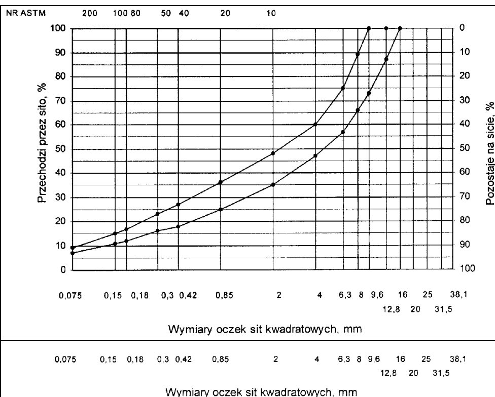
Rys. 7. Krzywe graniczne uziarnienia mieszanki mineralnej BA od 0 do 12,8 mm do warstwy ścieralnej nawierzchni drogi o obciążeniu ruchem od KR3 do KR6
