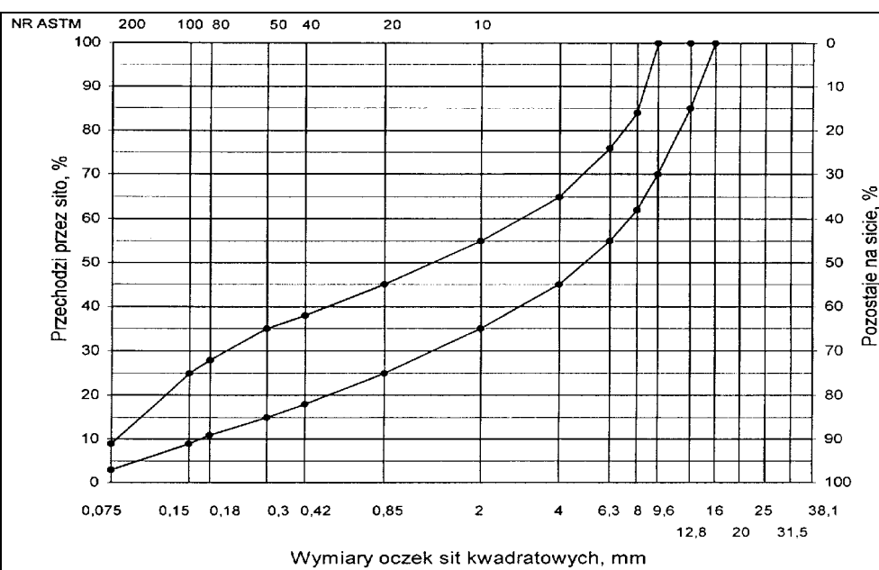
Rys. 10. Krzywe graniczne uziarnienia mieszanki mineralnej BA od 0 do 12,8 mm do warstwy wiążącej, wyrównawczej i wzmocniającej nawierzchni drogi o obciążeniu ruchem KR1 lub KR2
