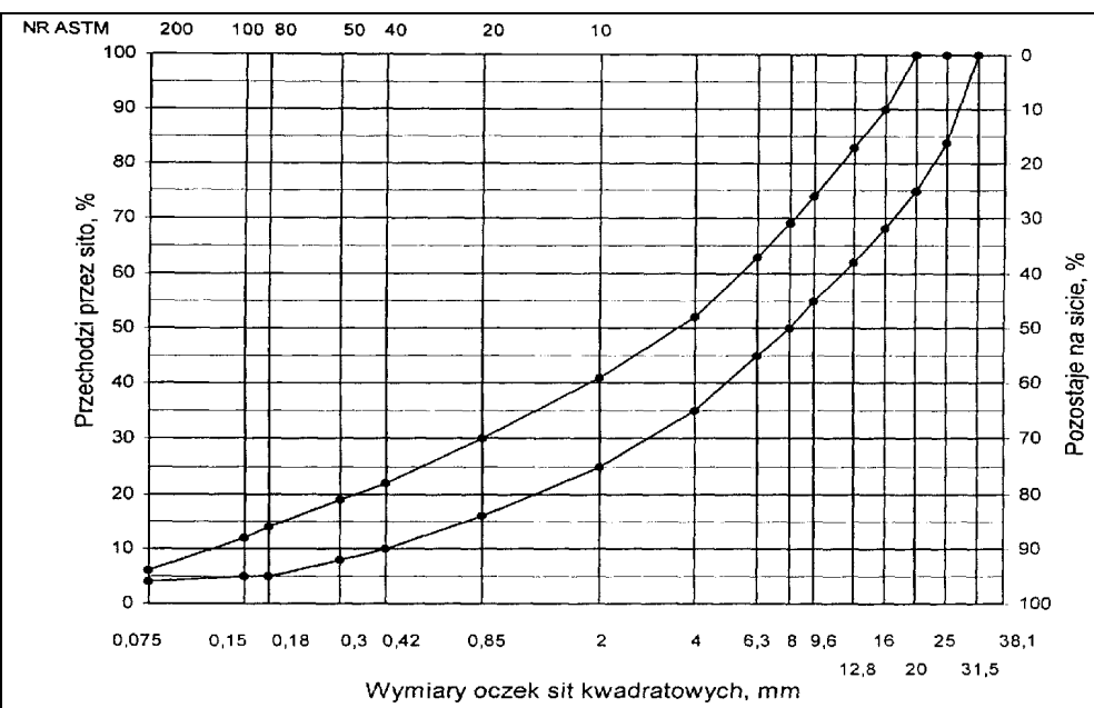
Rys. 11. Krzywe graniczne uziarnienia mieszanki mineralnej BA od 0 do 25 mm do warstwy wiążącej, wyrównawczej i wzmocniającej nawierzchni drogi o obciążeniu ruchem od KR3 do KR6
